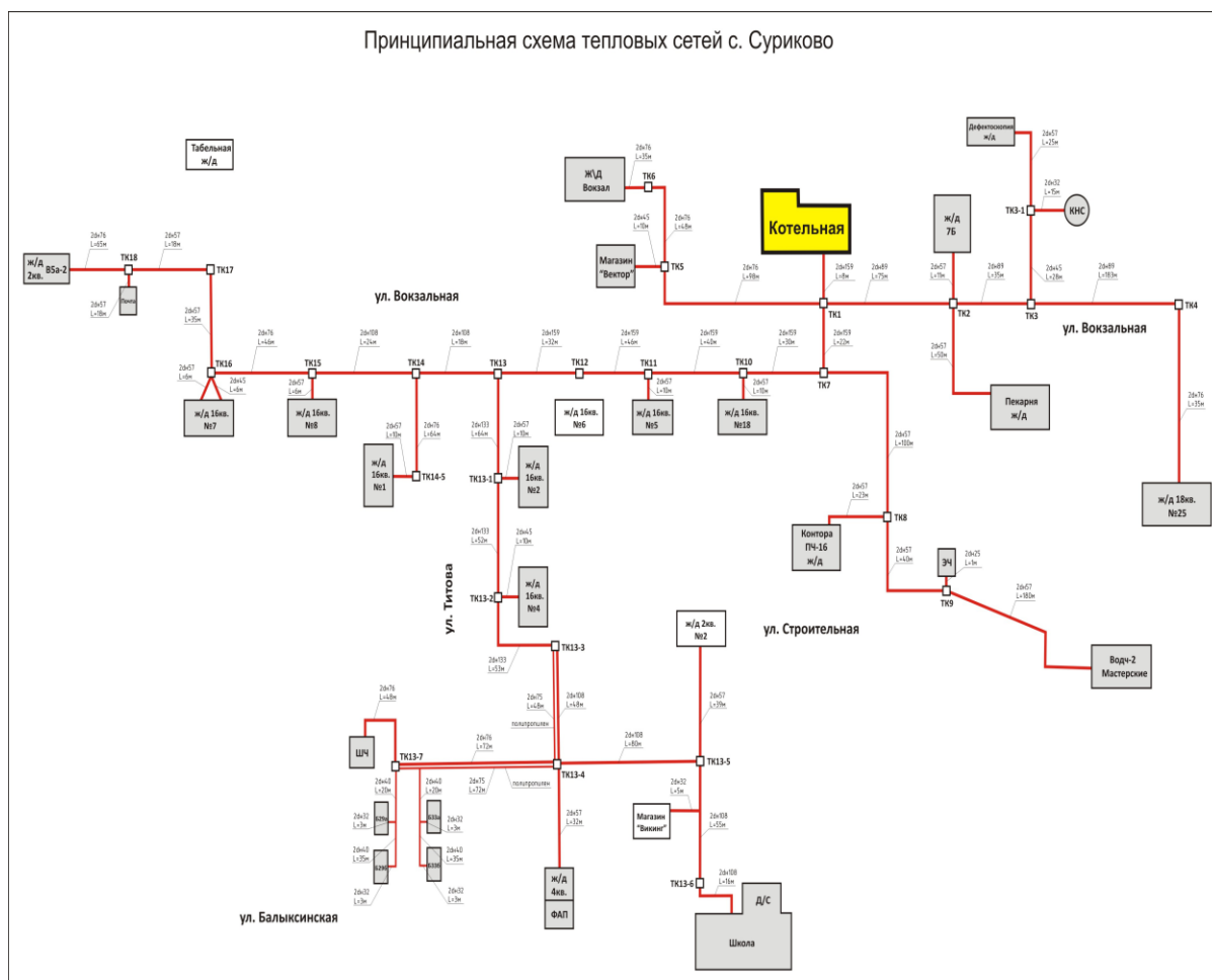
Рис. 1 Зона теплоснабжения
